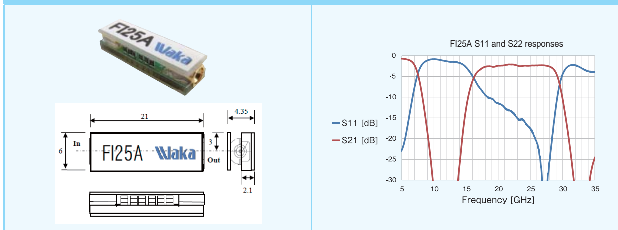
18-29 GHz Band Pass Filter (FI25A) (周波数 2 逡倍器出力の基本波成分抑制用)
