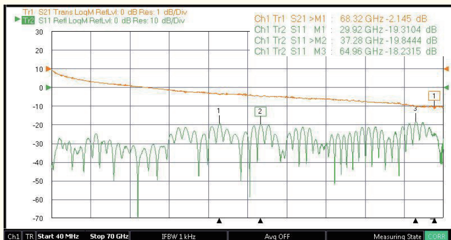
■データ (参考) SMPS/J-1.0mmW ケーブル Assy L=80mm
